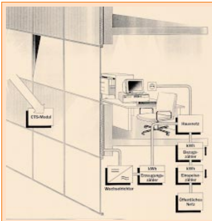
Photovoltaik: Die CTS-Modul-Fassade
