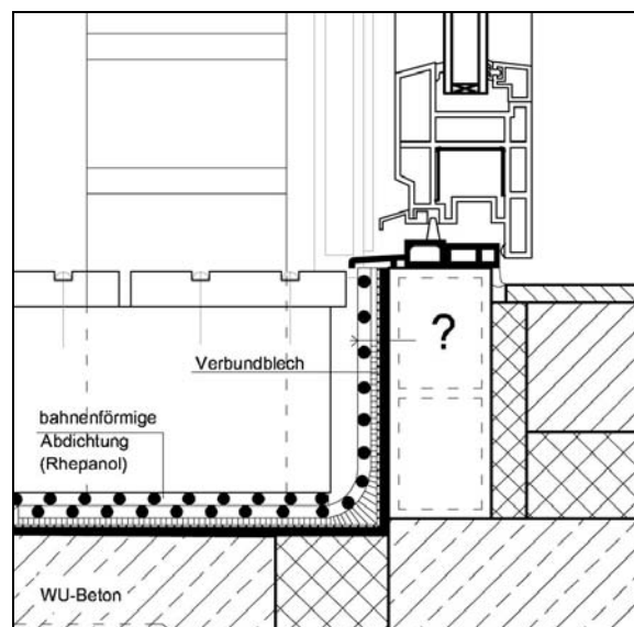
Abb. 2.5.6-5: Detailschnitt Balkonschwelle
