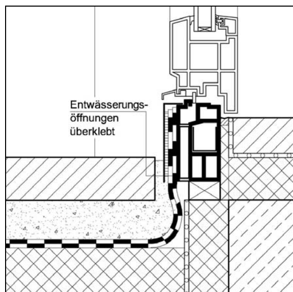
Abb. 2.3.6-4: Detail mangelhafter Terrassentüranschluss
