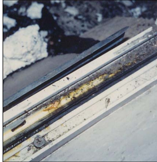
Abb. 2.3.6-2: Die Entwässerungsöffnungen im Rahmenprofil leiten Wasser hinter den mit Zinkblech abgedeckten Abdichtungsrand
