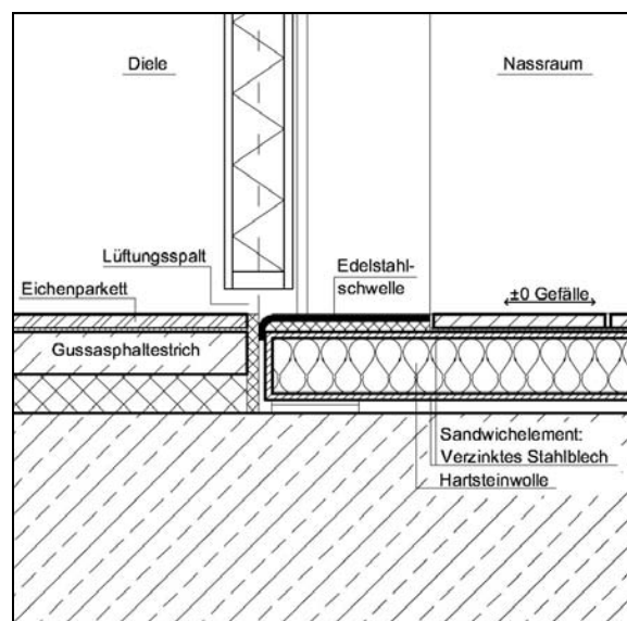
Abb. 3.3.2-5: mangelhaftes Detail Schwellenbereich zwischen Bad und Diele
