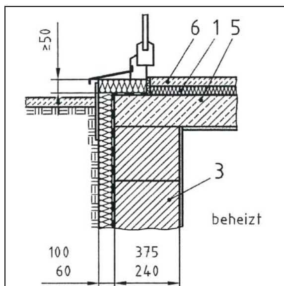
Abb. 2.1-4: Fenstertür, außengedämmtes Mauerwerk, Anschluss Terrasse [aus: DIN 4108 Bbl. 2:2006-03; Abb. 68] Legende: 1 Wärmedämmung (0,04 W/(mK)) 3 Mauerwerk ( 0,21 < \lambda \leq 1,1 W/(mK)) 5 Stahlbeton (2,3 W/(mK)) 6 Estrich
