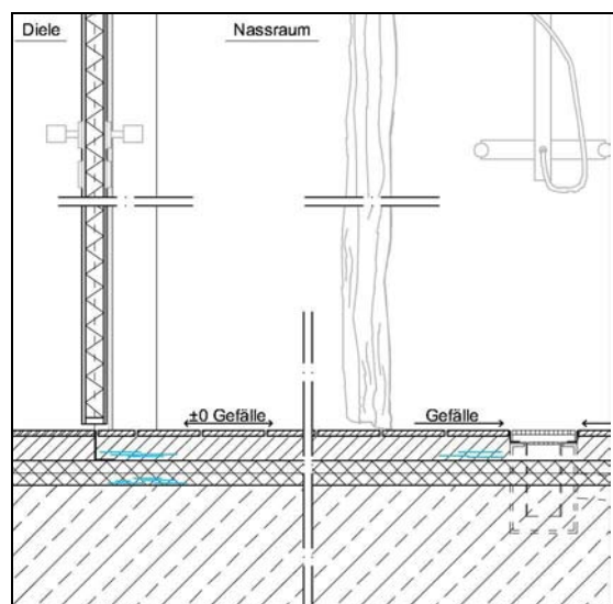
Abb. 3.3.1-3: Übersichtsskizze zur mangelhaften Nassraumabdichtung
