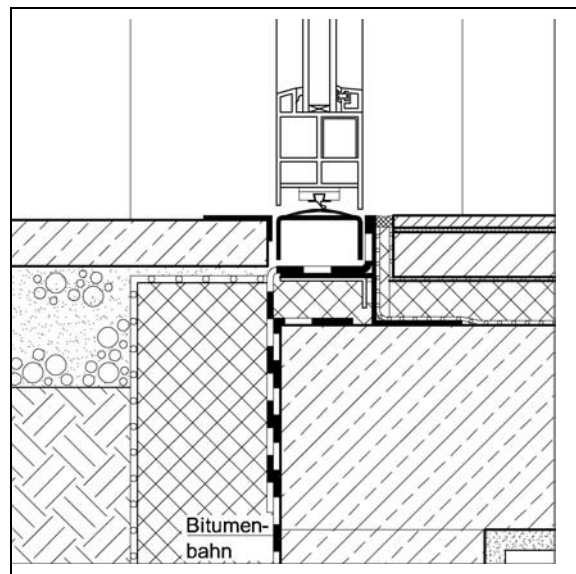
Abb. 2.6-7: Detailskizze Abdichtung Türschwelle
