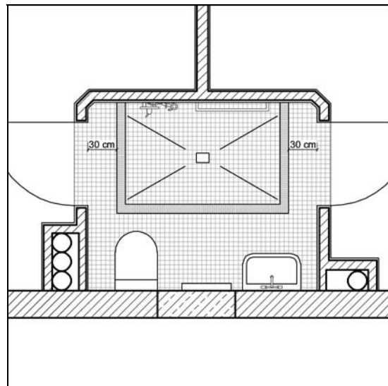
Abb. 3.5.1-3: Grundrisssskizze eines Duschbads für zwei Zimmer
