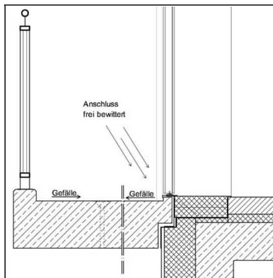
Abb. 2.3.5-3: Prinzipskizze mangelhafter Türanschluss
