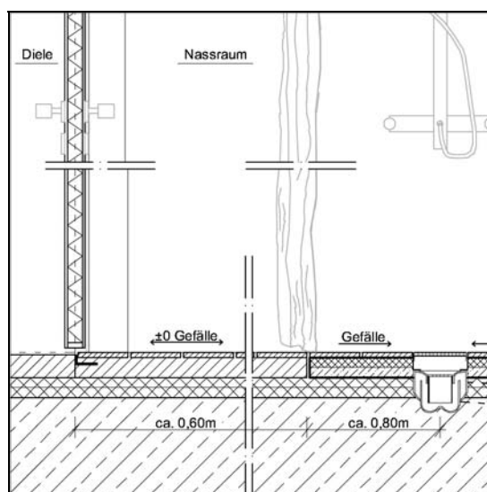
Abb. 3.5.3-3: Übersichtsskizze, Lage der Dusche
