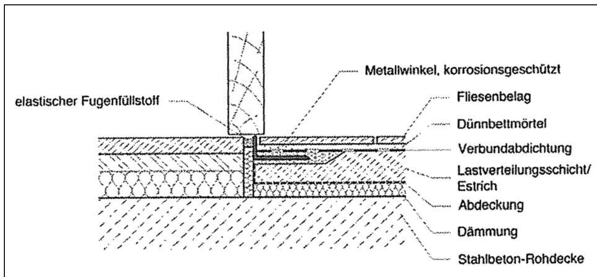
Abb. 3.2-3: Übergang im Türbereich (Beanspruchungsklasse AO) [ZDB Merkblatt, Januar 2010]
