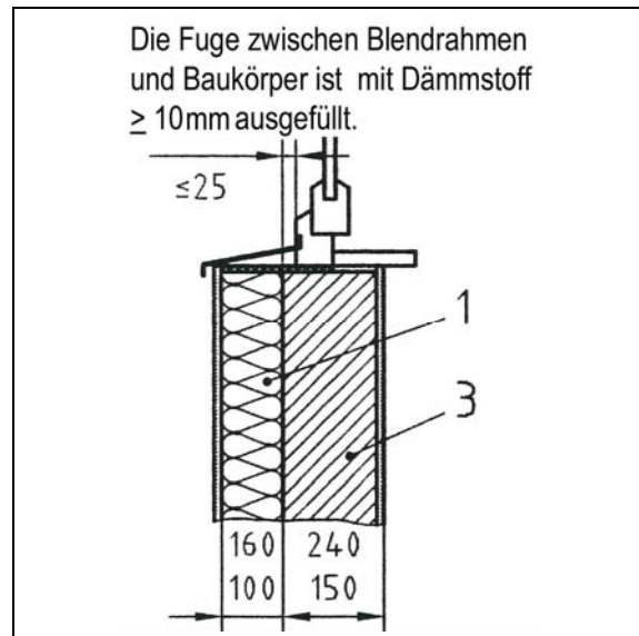
Abb. 2.1-7: Fensterbrüstung, außen gedämmtes Mauerwerk [aus: DIN 4108 Bbl. 2:2006-03; Abb. 43] Legende: 1 Wärmedämmung ( 0,04 \text{ W}/(\text{mK}) ) 3 Mauerwerk ( 0,21 < \lambda \leq 1,1 \text{ W}/(\text{mK}) )
