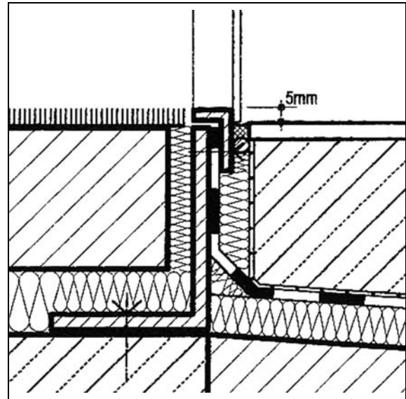
Abb. 3.6-4: Türschwelle Bad/Flur mit bahnenförmiger Abdichtung
