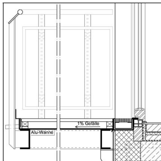
Abb. 2.5.7-3: Detail Balkonanschluss
