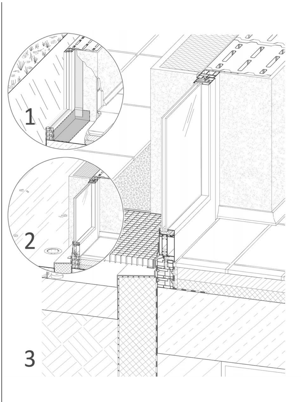
Abb. 2.6-3: Innenansicht: Aufkantung der Abdichtung auf der Außenseite der Tür, Terrassenanschluss mit Wärmedämmverbundsystem
