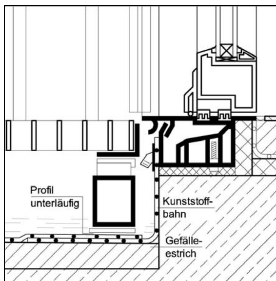
Abb. 2.5.1-5: Detail: Anschluss Balkon/Türschwelle
