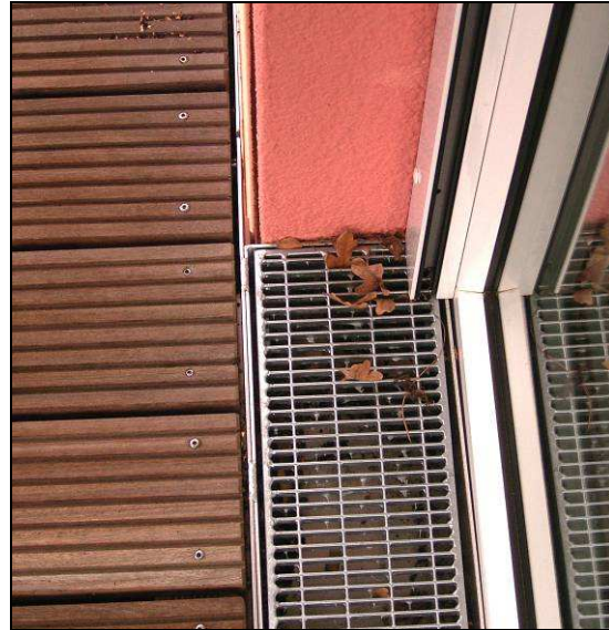
Abb. 2.5.7-2: Detail Türschwelle
