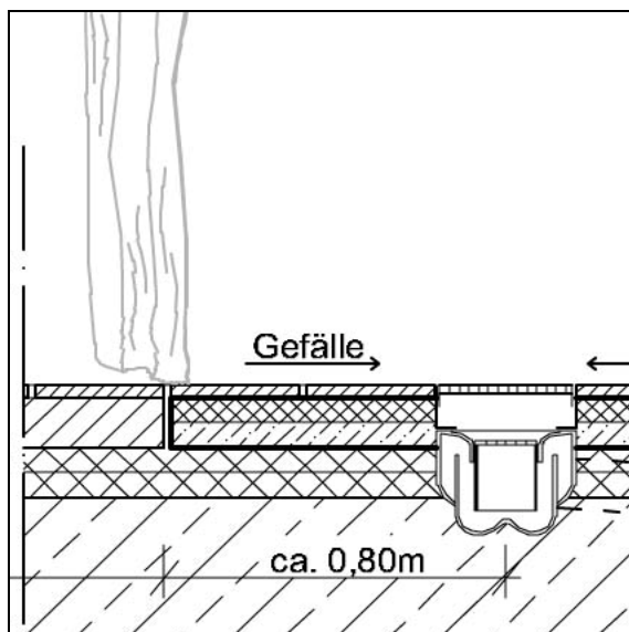
Abb. 3.6-2: Vorgefertigtes Unterbauelement im Duschbereich
