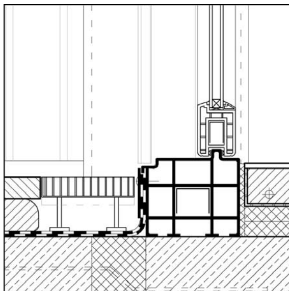
Abb. 2.3.1-5: Detail: mangelhafter Abdichtungsanschluss an die Schiebetür und im Bereich der Türleibung
