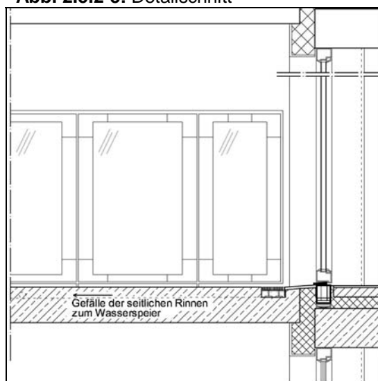
Abb. 2.5.2-3: Detailschnitt
