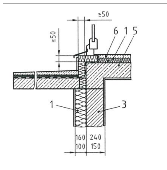
Abb. 2.1-5: Fenstertür, außengedämmtes Mauerwerk, Anschluss Balkonplatte [aus: DIN 4108 Bbl. 2:2006-03; Abb. 70] Legende: 1 Wärmedämmung (0,04 W/(mK)) 3 Mauerwerk ( 0,21 < \lambda \leq 1,1 W/(mK)) 5 Stahlbeton (2,3 W/(mK)) 6 Estrich
