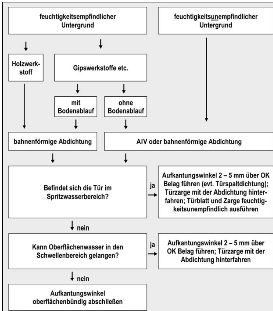
Abb. 4.6-1: Flussdiagramm zu den erforderlichen Abdichtungsmaßnahmen auf Bodenflächen mit niveaugleichen Duschen bei mäßiger Beanspruchung
