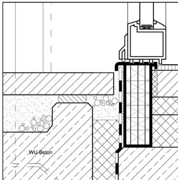
Abb. 2.5.5-5: Detailschnitt Wohnungseingangstür
