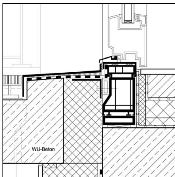
Abb. 2.5.2-10: Höhenunterschied ca. 2 cm
