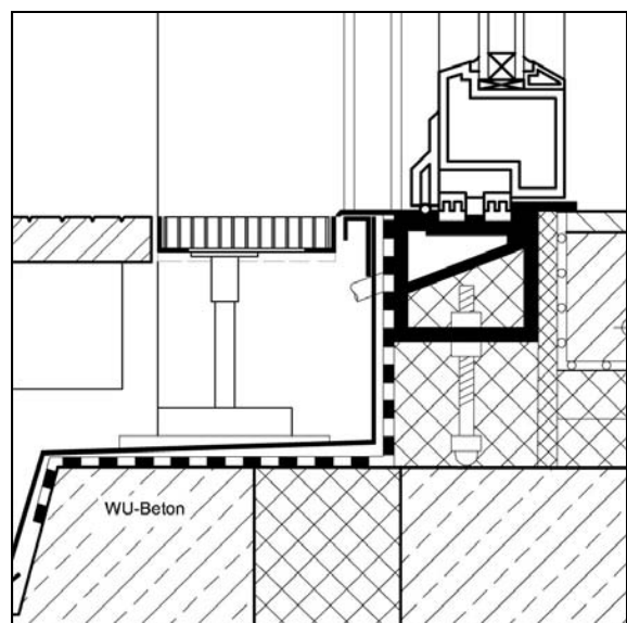
Abb. 2.5.3-5: Detailschnitt im Bereich der Türschwelle
