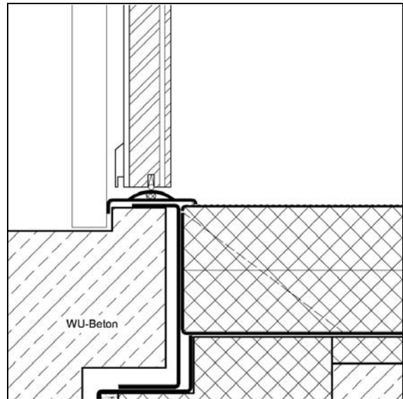
Abb. 2.3.5-5: Detailschnitt im Bereich der mangelhaft ausgeführten Türschwelle
