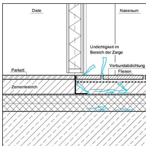
Abb. 3.3.1-4: Übergangsbereich zur Diele, Estrich ist durch einen Stellwinkel getrennt.
