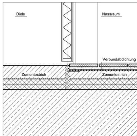
Abb. 3.5.3-5: Detailschnitt Türschwelle
