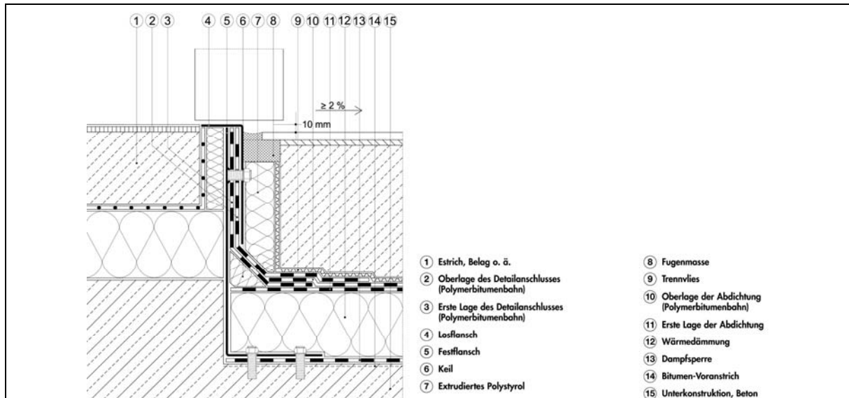
Abb. 2.1-3: Türanschluss mit Polymerbitumenbahnen, barrierefrei [aus: [VDD 2007]]
