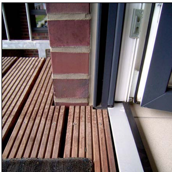
Abb. 2.5.6-4: Zugangssituation vom Wohnzimmer auf den Balkon
