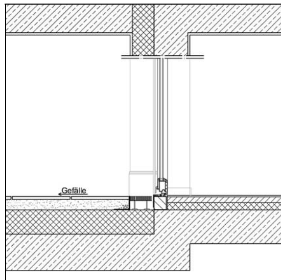
Abb. 2.5.8-3: Detailskizze Türschwelle/Dachterrasse
