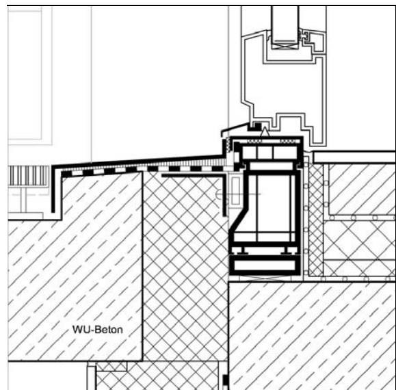
Abb. 2.5.2-5: Detailskizze Anschlusssituation Türschwelle
