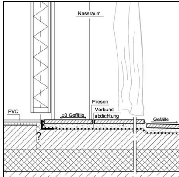
Abb. 3.5.1-5: Detailschnitt Dusche / Tür
