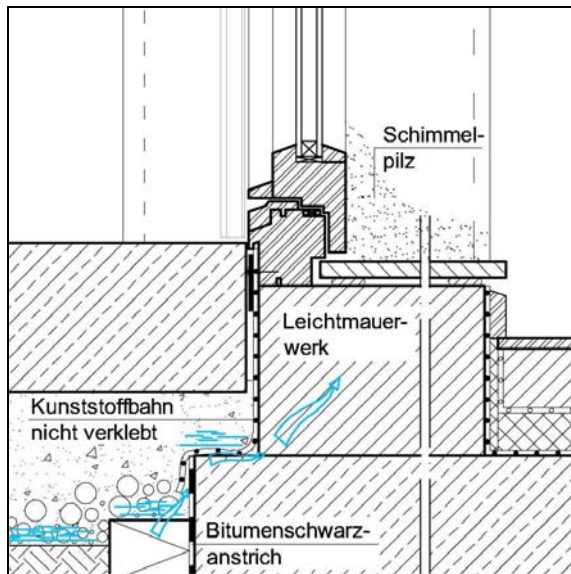
Abb. 2.3.3-4: Detailskizze Türanschluss
