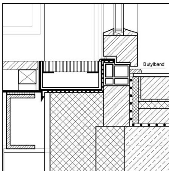
Abb. 2.5.7-5: Detailschnitt Balkonschwelle
