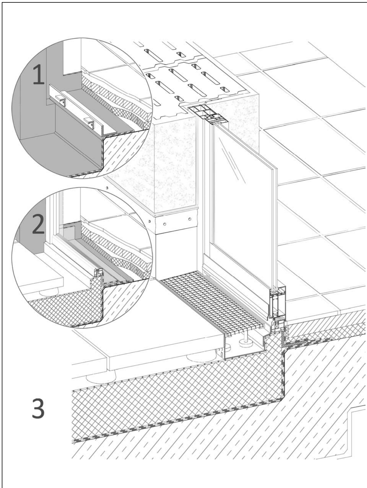
Abb. 2.6-4: Außenansicht: Aufkantung der Abdichtung auf der Innenseite der Tür, Umkehrdach und verputztes Mauerwerk
