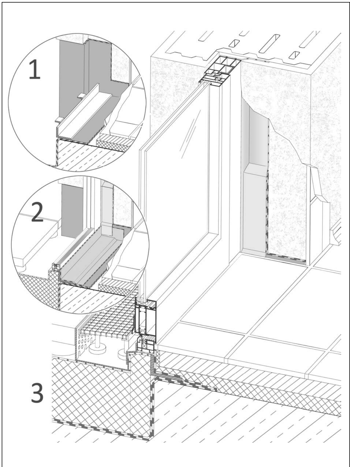
Abb. 2.6-5: Innenansicht: Aufkantung der Abdichtung auf der Innenseite der Tür, Umkehrdach und verputztes Mauerwerk
