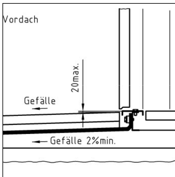
Abb. 2.1-2: Abschluss an Türschwelle; barrierefrei, nicht drückendes Wasser; hohe Beanspruchung; (Parkdeck, Bahnenabdichtung mit Gussasphalt) [aus: DIN 18195 Bbl.1,2006-01, Bild 17]
