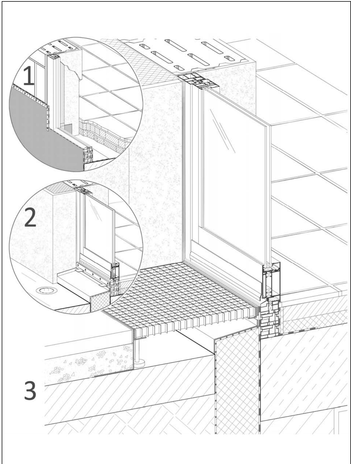
Abb. 2.6-2: Außenansicht: Aufkantung der Abdichtung auf der Außenseite der Tür, Terrassenanschluss mit Wärmedämmverbundsystem; kein Versprung der Abdichtungsebene
