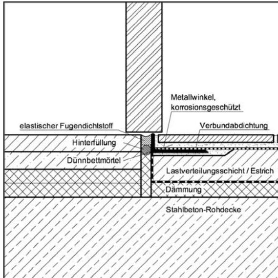
Abb. 3.6-3: Türschwelle Bad/Flur mit Verbundabdichtung
