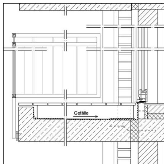
Abb. 2.5.6-3: Prinzipskizze Balkonanschluss / Türschwelle
