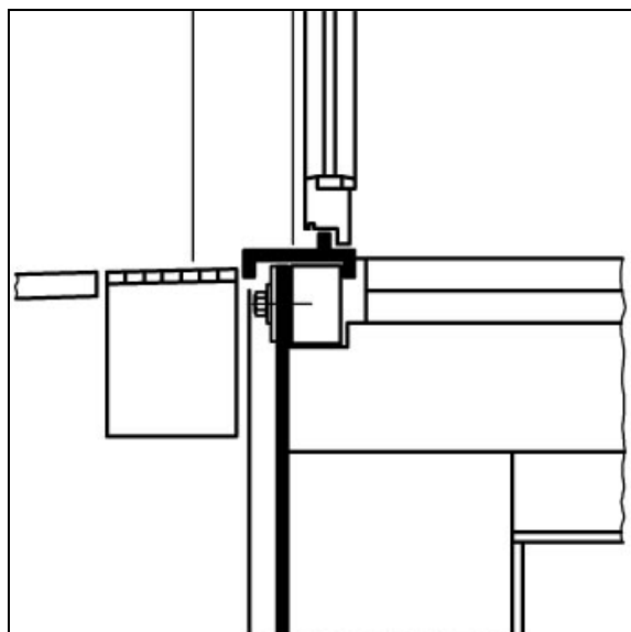
Abb. 2.1-1: Sockel-Türanschluss, niveaugleich [aus: DIN 18195 Bbl.1, 2006-01, Bild 10]
