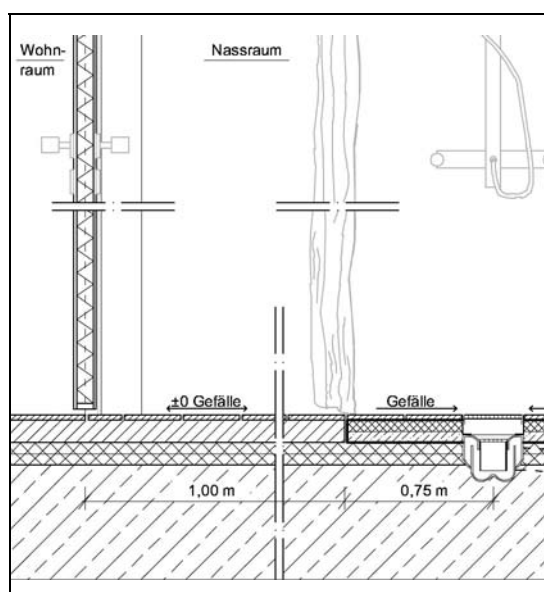
Abb. 3.5.2-3: Detail Türschwelle, keine Trennung der Bodenflächen
