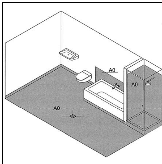
Abb. 3.2-2: Häusliches Bad mit Badewanne ohne Duschnutzung und mit Bodenablauf [ZDB-Merkblatt Verbundabdichtungen, Januar 2010]
