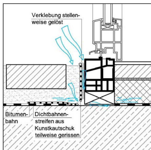
Abb. 2.3.2-5: Detail: mangelhafter Abdichtungsanschluss an das Schwellenprofil der Hauseingangstür
