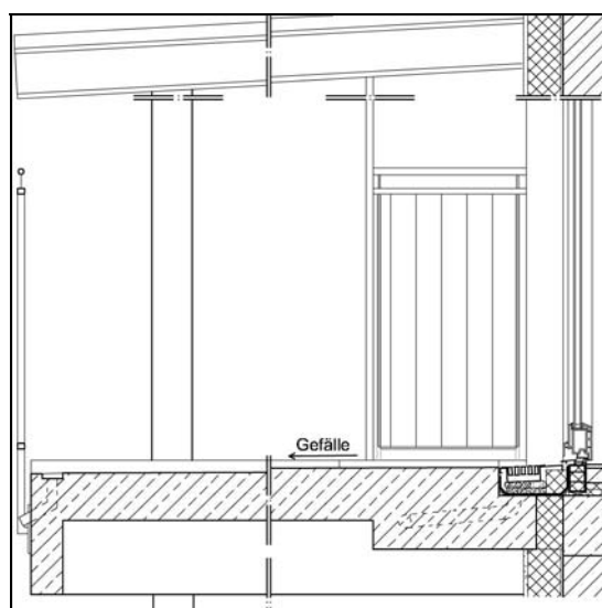
Abb. 2.5.4-3: Schwelkenanschluss
