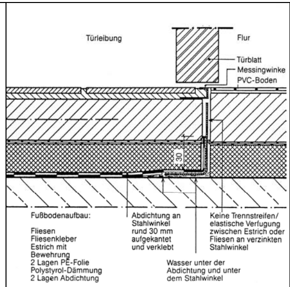
Abb. 3.3.3-5: Schnitt im Bereich der mangelhaft ausgeführten Türschwelle
