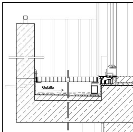
Abb. 2.5.1-3: Prinzipskizze, Detailschnitt Balkon
