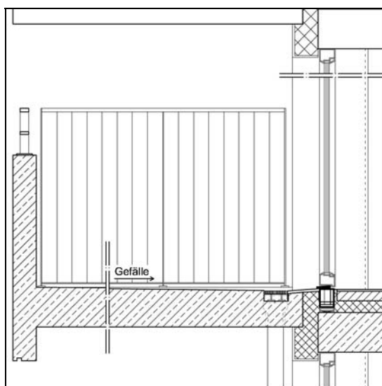
Abb. 2.5.2-8: Schnitt Balkon / Türschwelle
