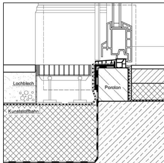
Abb. 2.5.8-5: Detailskizze Türschwelle/Dachterrasse
