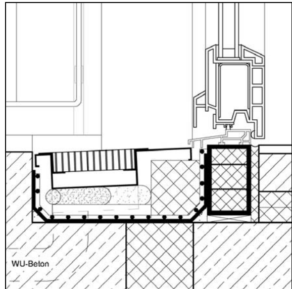
Abb. 2.5.4-5: Detailschnitt Türschwelle Laubengang
