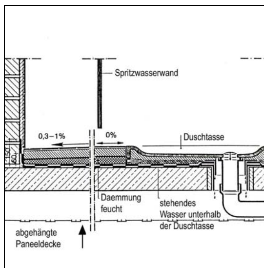
Abb. 3.3.3-3: Übersichtsskizze: Schnitt durch den mangelhaften Fußbodenaufbau
