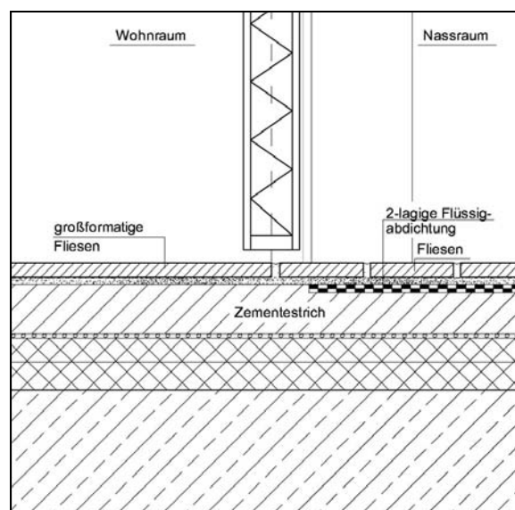
Abb. 3.5.2-5: Detailschnitt Türschwelle
