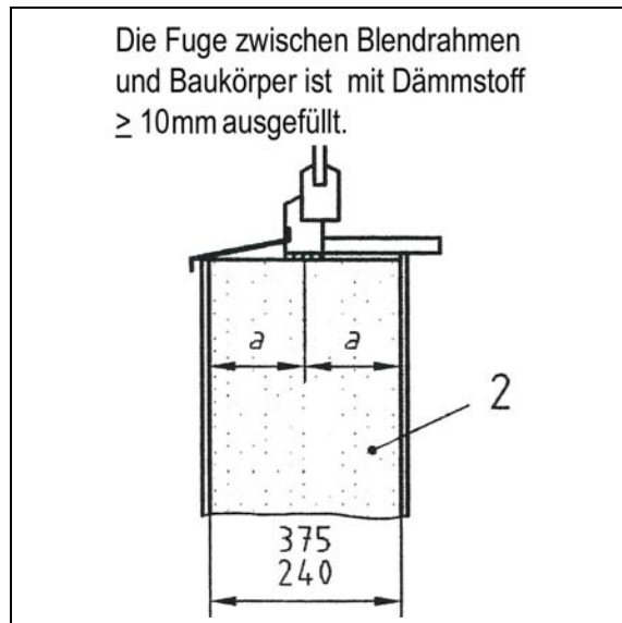
Abb. 2.1-6: Fensterbrüstung, monolithisches Mauerwerk [aus: DIN 4108 Bbl. 2:2006-03; Abb. 42] Legende: 2 Mauerwerk ( \leq 0,21 \text{ W}/(\text{mK}) )
