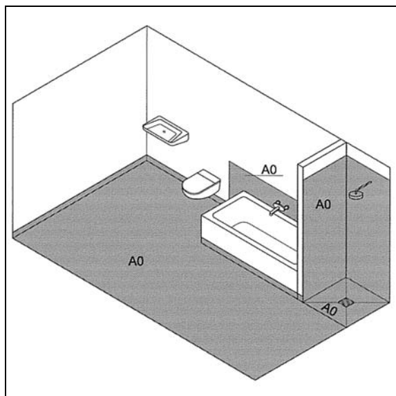
Abb. 3.2-1: Häusliches Bad mit Badewanne ohne Duschnutzung und mit Bodenablauf im Duschbereich [ZDB-Merkblatt Verbundabdichtungen, Januar 2010]
