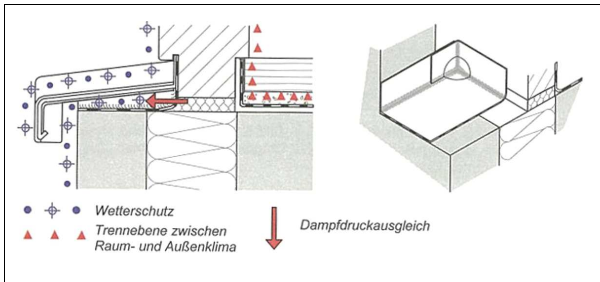
Abb. 2.6-1: Unterer Anschluss im Bereich der äußeren Fensterbank mit einer diffusionsoffenen Dichtfolie zum Dampfdruckausgleich nach außen, im Eckbereich wannenförmig ausgebildet. [aus: Leitfaden zur Montage, RAL, Dezember 2006, Abb. 6.12]
