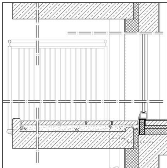
Abb. 2.5.5-3: Prinzipskizze: Schnitt Wohnungseingangstür
