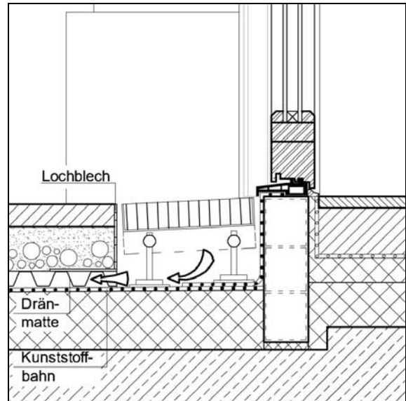
Abb. 2.3.4-5: Detail mangelhafter Schwellenanschluss
