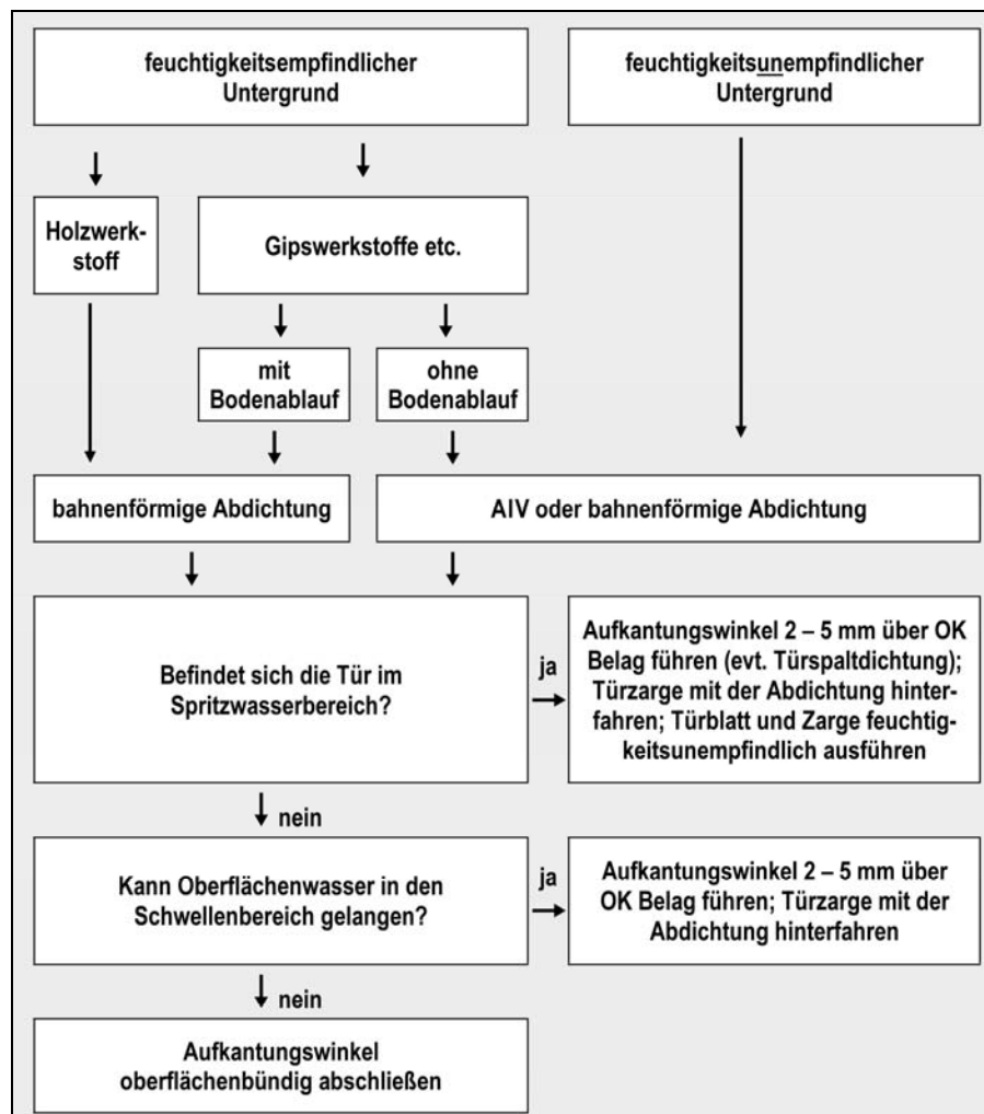
Abb. 3.6-4: Flussdiagramm zu den erforderlichen Abdichtungsmaßnahmen auf Bodenflächen mit niveaugleichen Duschen bei mäßiger Beanspruchung
